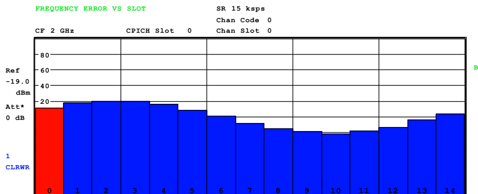
Bild 48 Relativer Frequenzfehler über Slot
