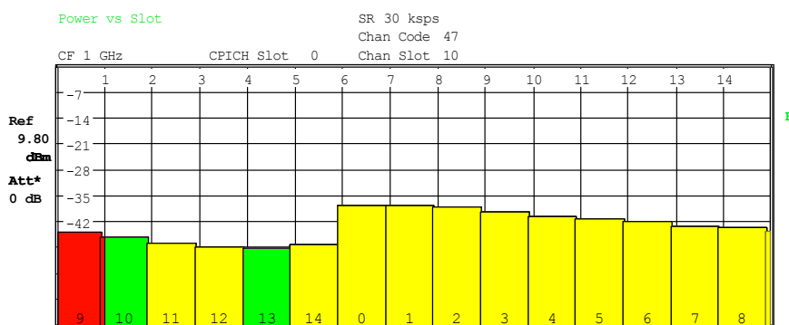
Bild 29 Power versus Time für einen Kanal mit fehlerhaften Pilot-Symbolfolgen
