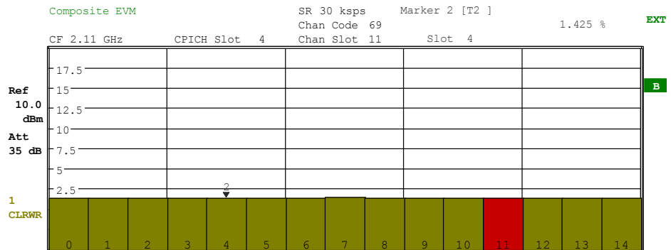
Bild 18 Darstellung des Composite EVM - alle im Signal enthaltenen Kanäle als aktiv erkannt
