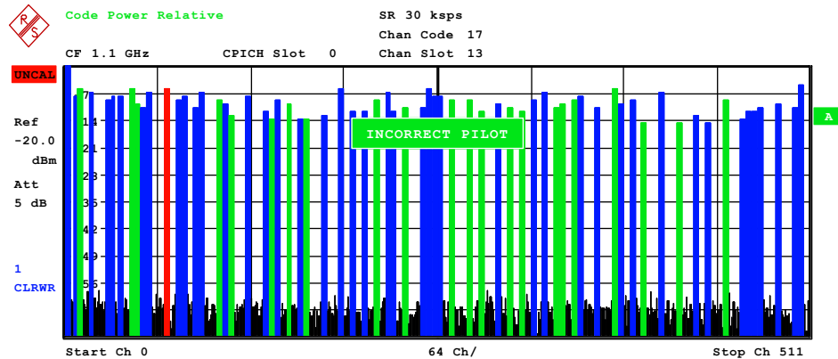
Bild 16 Code-Domain-Power-Diagramm mit inkorrekten Pilot-Symbolen
