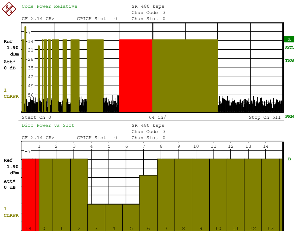
Bild 60 Code Domain Power und Power Versus Slot eines Compressed Channel
