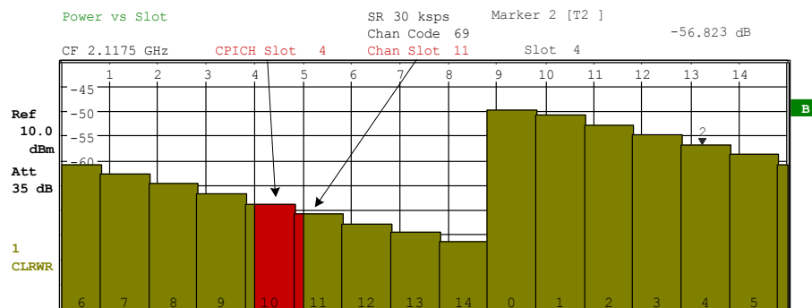
Bild 28 Power versus Slot für einen belegten Kanal mit einem Timing-Offset von 22528 Chips
