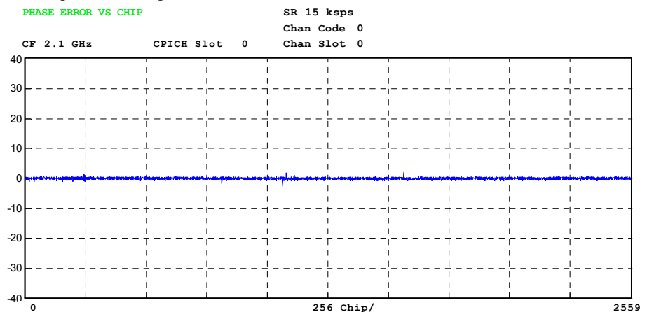
Bild 25 Darstellung des Phasenfehlers über Chip
