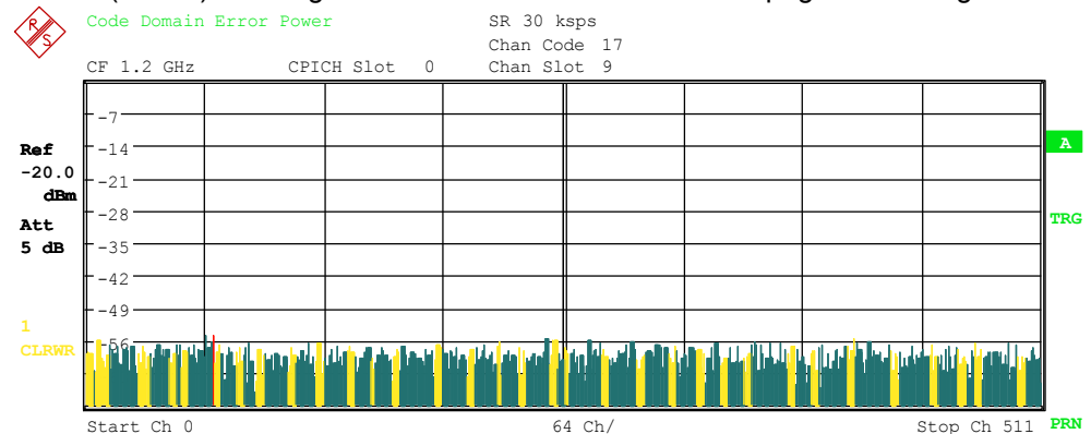
Bild 32 Darstellung des Code Domain Error eines fehlerfreien Signals
