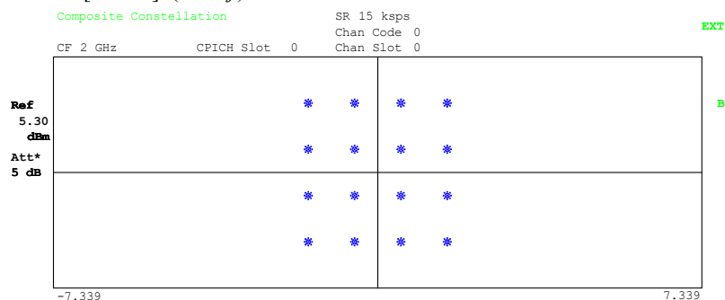
Bild 31 Darstellung des Composite Constellation-Diagramms
