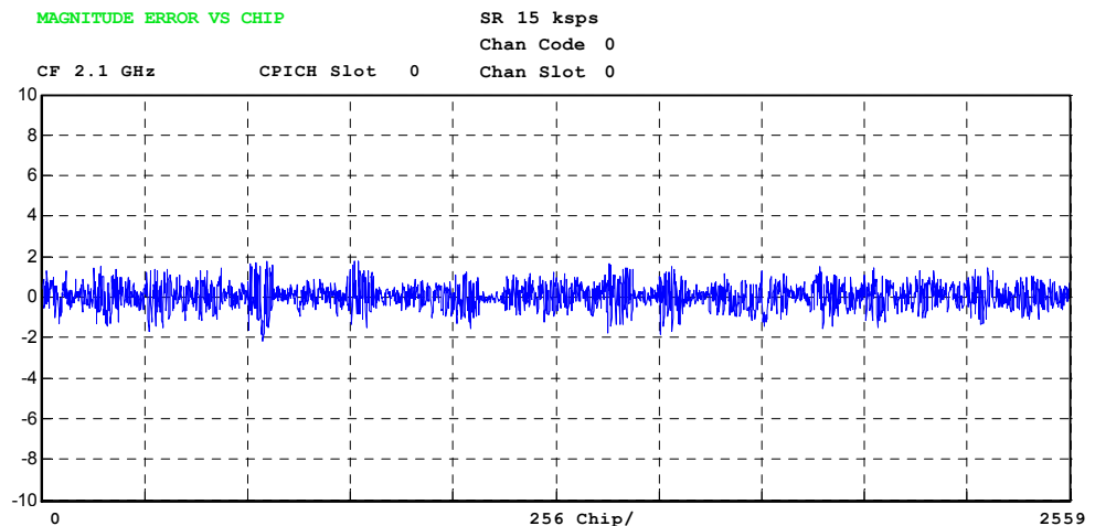
Bild 23 Darstellung der Messung Magnitude Error versus Chip
