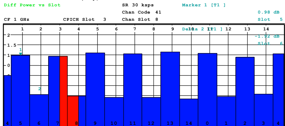
Bild 65 Slot-Leistungsdifferenz einer wechselnden Slot- Leistungs-Sequenz, mit Leistungsschritten von 1 dB zwischen jeder Stufe
