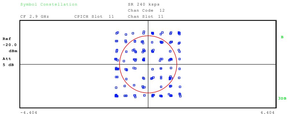
Bild 40 Darstellung des Symbol Constellation Diagramms für 64QAM
