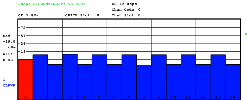
Bild 49 Phasensprung über Slot
