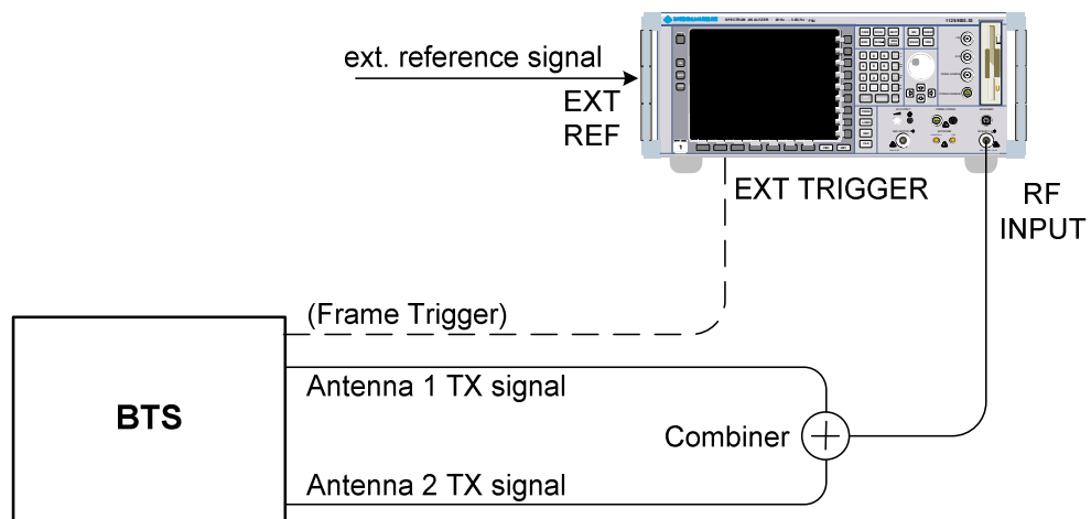
Bild 11 Aufbau für Time-Alignment-Error-Messung
