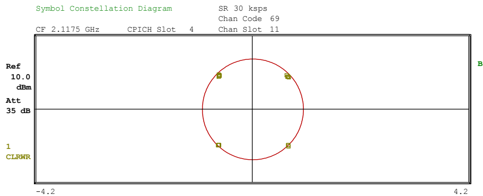
Bild 39 Darstellung des Symbol Constellation Diagramms
