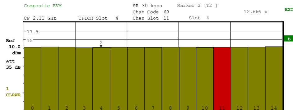
Bild 19 Darstellung des Composite EVM – ein Kanal nicht als aktiv erkannt
