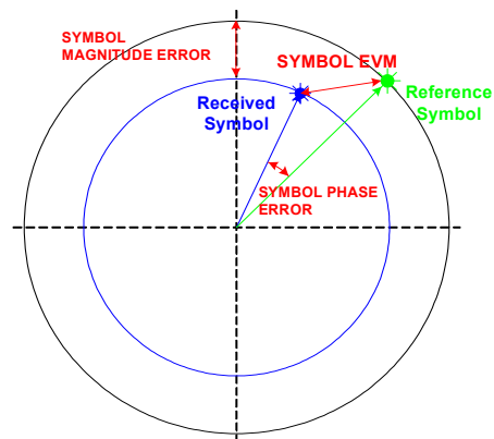
Bild 43 Schematische Darstellung von Referenz- und Empfangssymbol zur Berechnung des Symbolphasenfehlers
