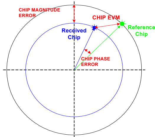
Bild 24 Schematische Darstellung des Referenzsignalchips und des Chips des empfangenen Signals zur Berechnung von Betrag, Phase und Vektorfehler.
