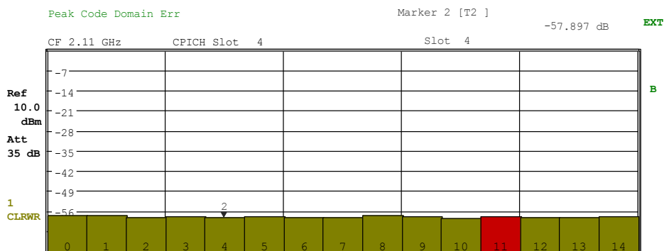
Bild 20 Peak Code Domain Error – alle im Signal enthaltenen Kanäle als aktiv erkannt
