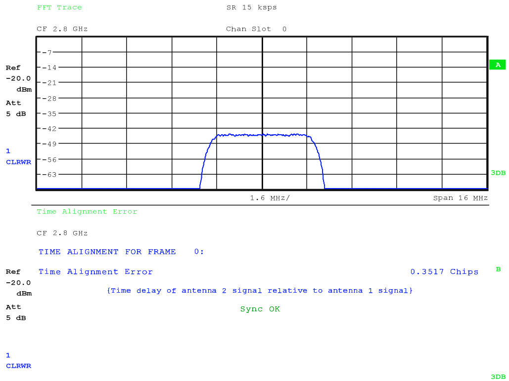
Bild 12 Ergebnisanzeige der Time-Alignment-Error-Messung
