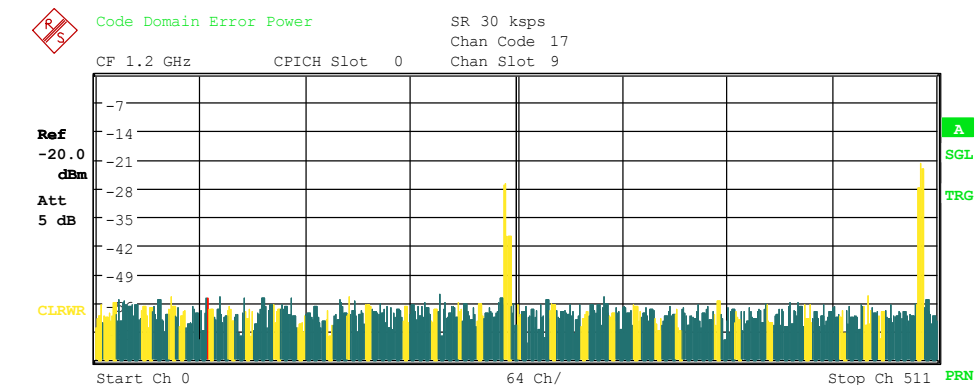
Bild 33 Darstellung des Code Domain Errors eines fehlerbehafteten Signals
