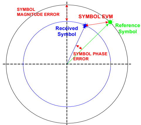
Bild 44 Schematische Darstellung von Referenz- und Empfangssymbol zur Berechnung des Amplitudenfehlers der Symbole
