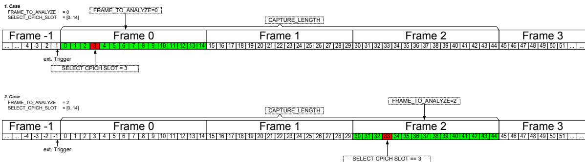
Bild 66 Datenstruktur des gemessenen und analysierten Frames
