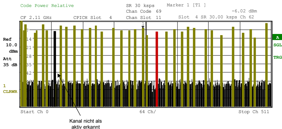
Bild 15 Code-Domain-Power-Diagramm mit einem nicht erkannten Kanal
