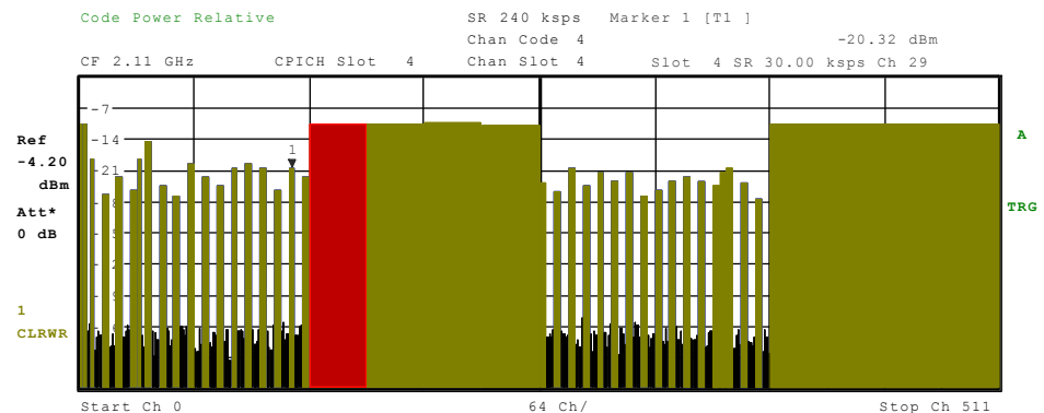
Bild 17 Code-Domain-Power-Diagramm, Test-Modell 5
