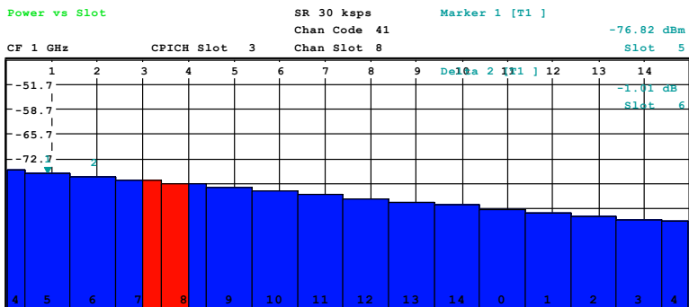
Bild 55 Absolute Slot-Leistung bei abfallender Slot Leistung
