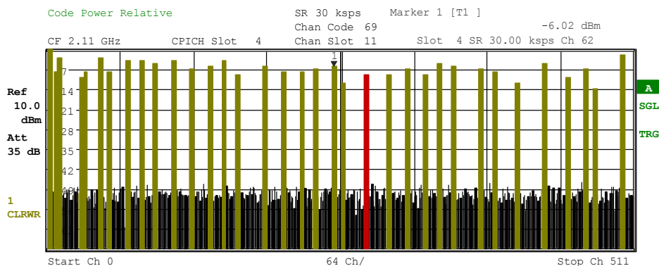
Bild 14 Code-Domain-Power-Diagramm, alle Kanäle als aktiv erkannt
