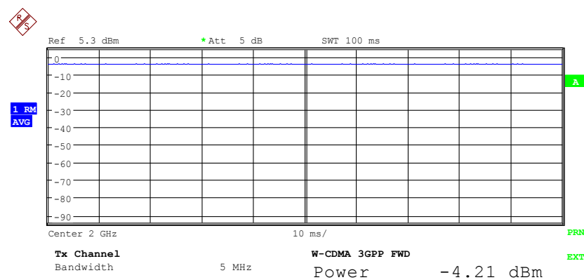
Bild 4 Messung der Leistung im 3.84-MHz-Übertragungskanal
