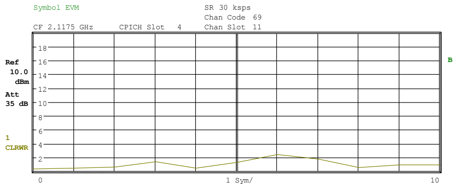
Bild 41 Error Vector Magnitude für einen Slot eines Kanals
