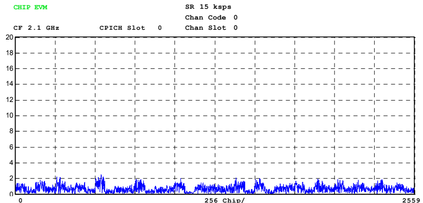
Bild 22 Darstellung des Vektorfehlers der Messung EVM versus Chip
