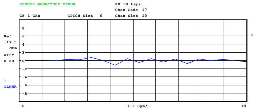
Bild 42 Darstellung Amplitudenfehler der Symbole
