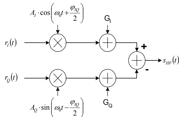
Bild 27 Grundmodell möglicher IQ-Impairment-Parameter in komplexen Aufwärtsumsetzern.
