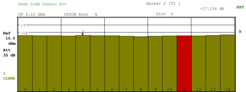
Bild 21 Peak Code Domain Error – ein Kanal nicht als aktiv erkannt
