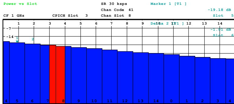
Bild 54 Relative Slot-Leistung bei abfallender Slot Leistung.
